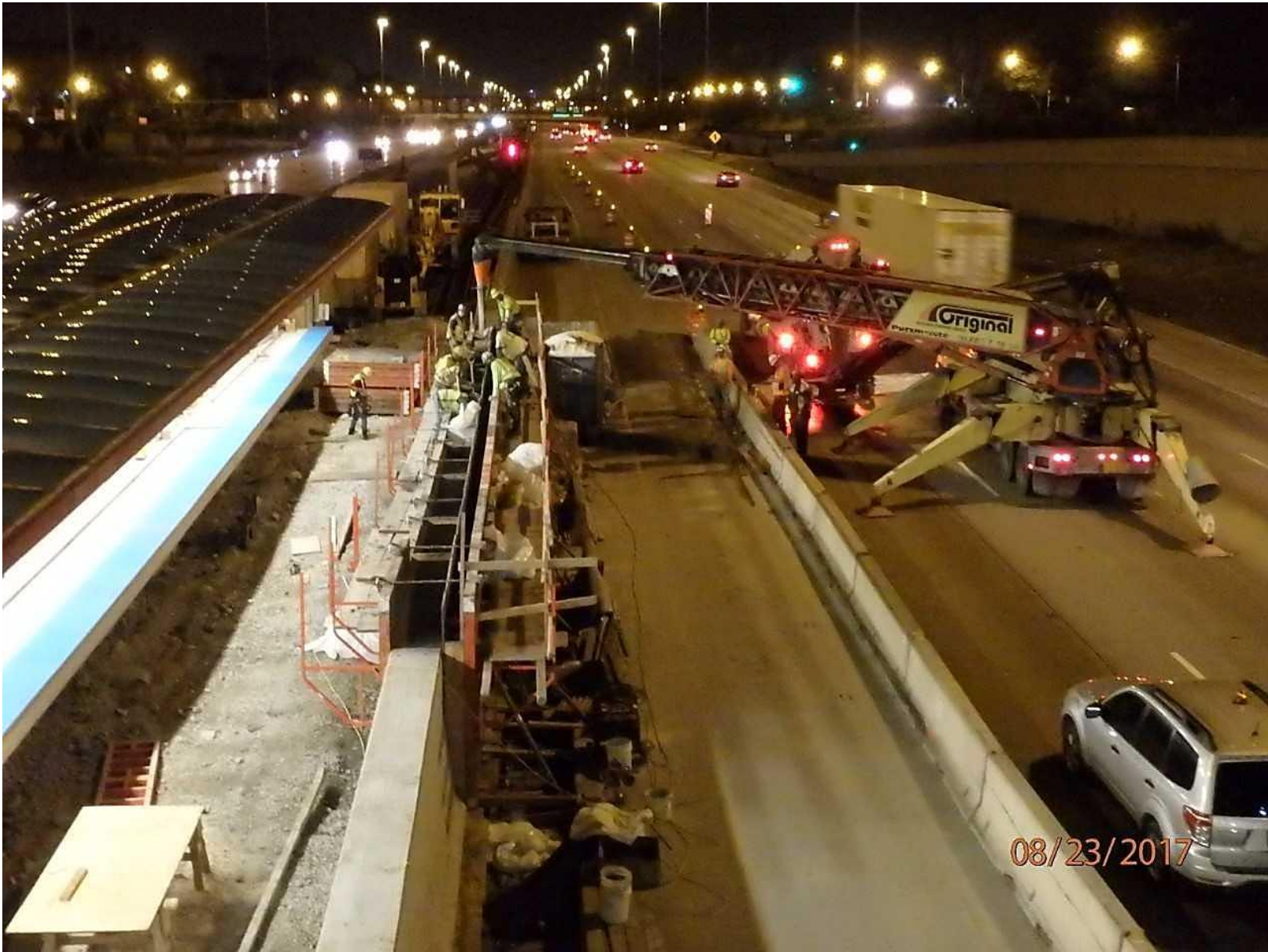
Concrete Pour - North Terminal East Side Crash Barrier Wall
